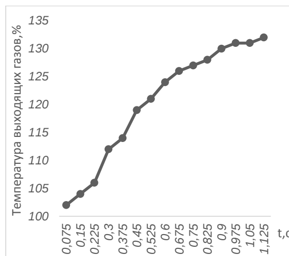
Рис.4. Изменение температуры выходящих газов во время помпажа [2]
