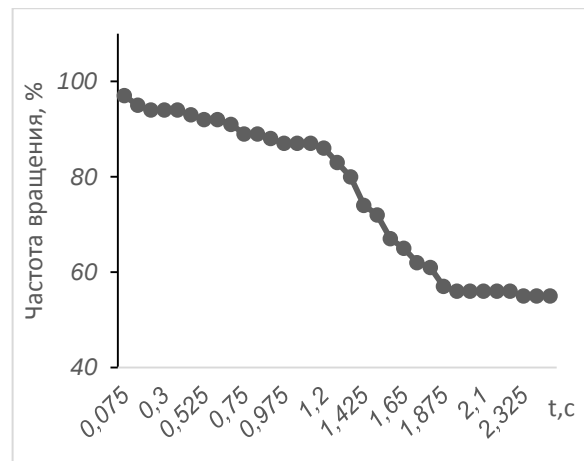
Рис.3. Динамика частоты вращения ротора турбины ГТД во время помпажа [2]
