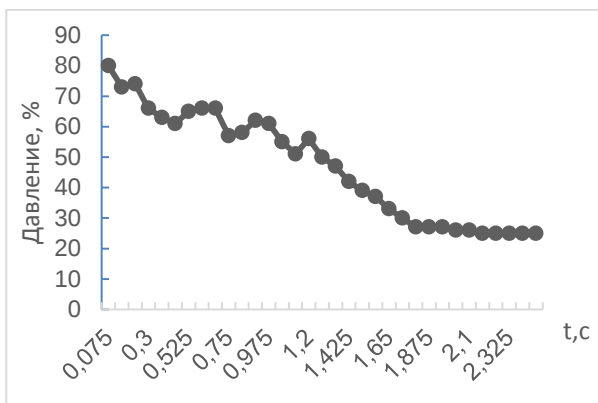
Рис.1. Изменение давления за компрессором во время помпажа [2]
