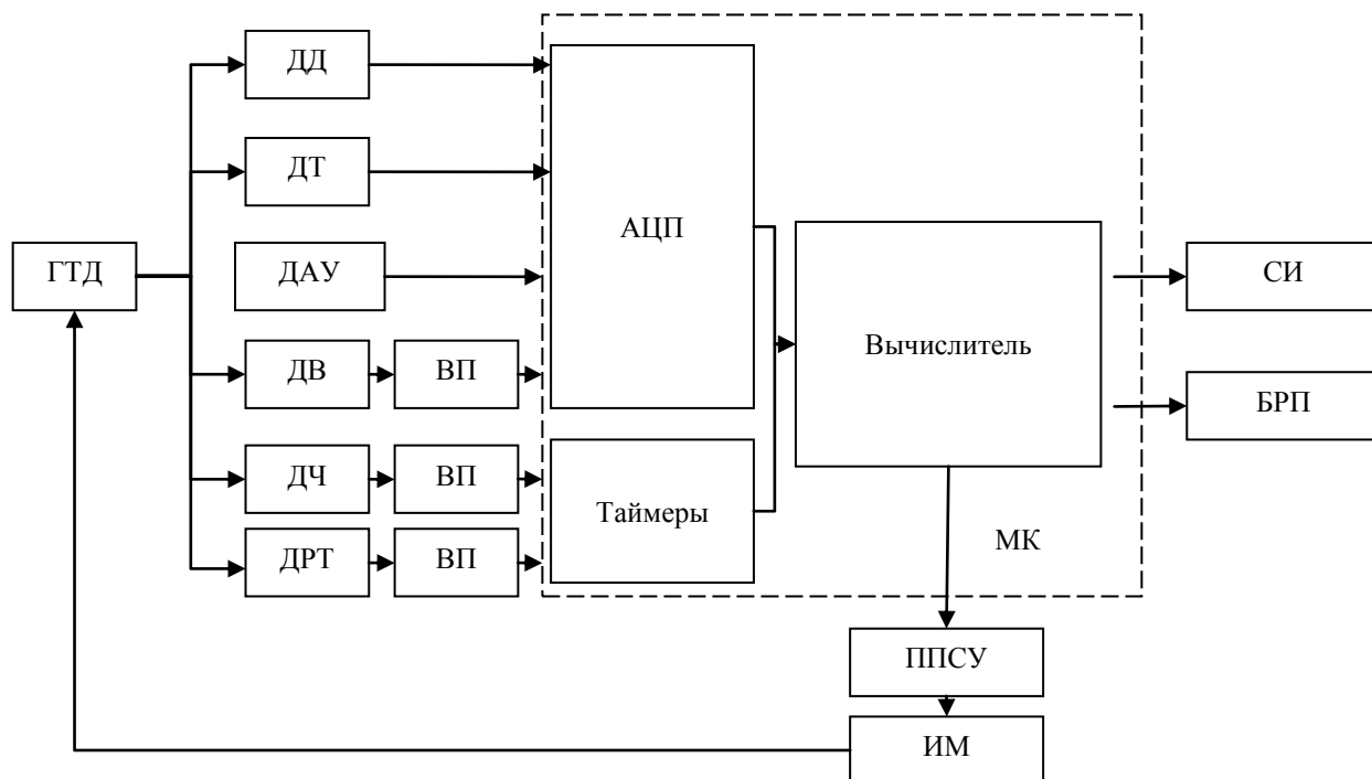
Рис.5. Структурная схема системы диагностики предпомпажного состояния ГТД [11]:
