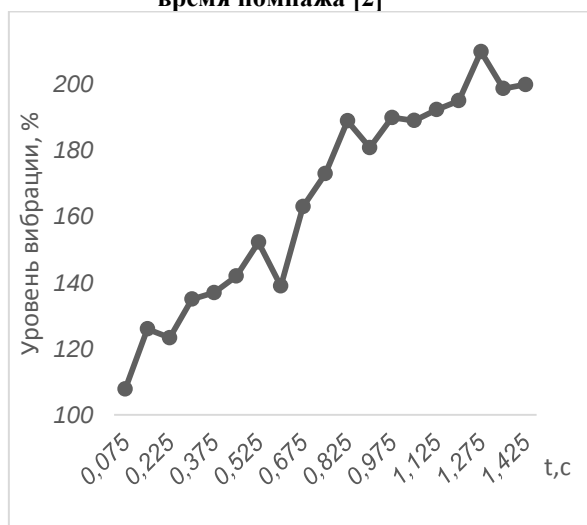
Рис.2. Изменение уровня вибрации во время помпажа
